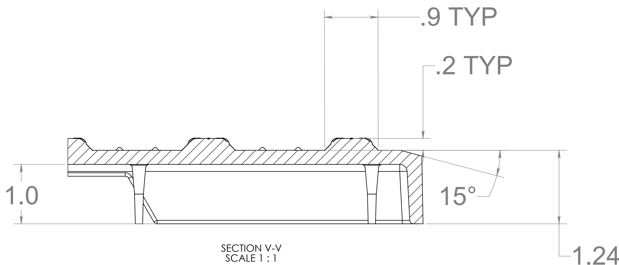
SECTION V-V SCALE 1:1
